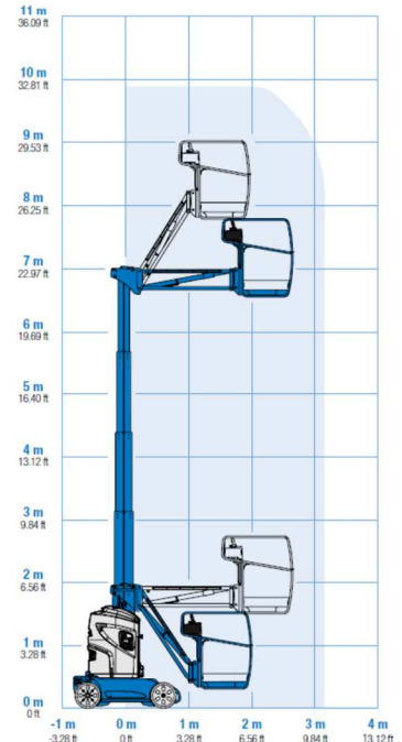
Diagrama de trabajo GR-26 J
