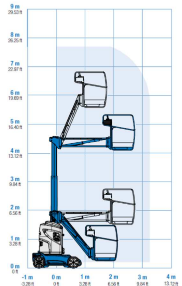
Diagrama de trabajo GR-26 J
